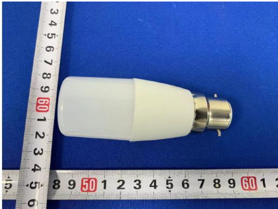
Fig. 3 (Lamp cap type: B22(d))
